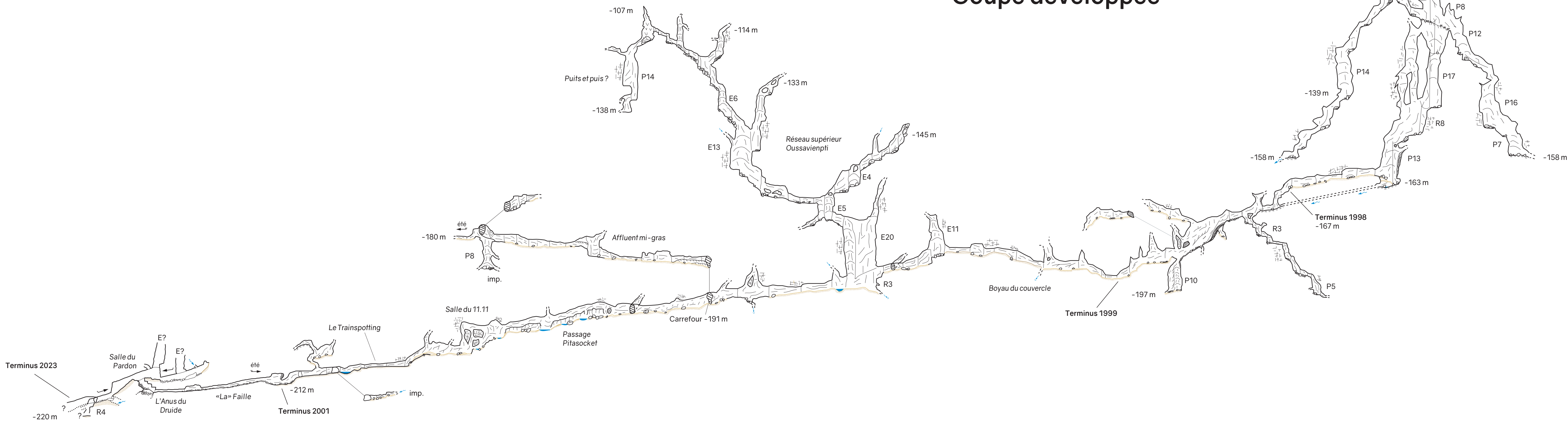
Coupe développée
